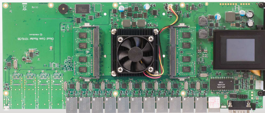
CCR1016-12G-BU
